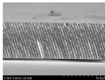
图 4 倾斜光栅扫描电镜图像
