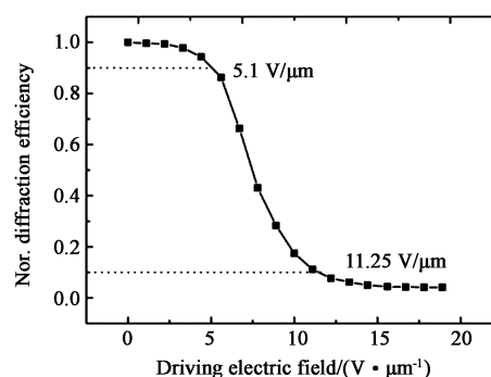
图 8 归一化衍射效率随场强的变化关系曲线
