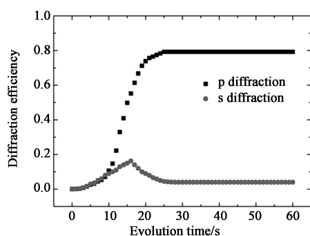
图 3 倾斜液晶/聚合物光栅衍射效率随时间演化特性
