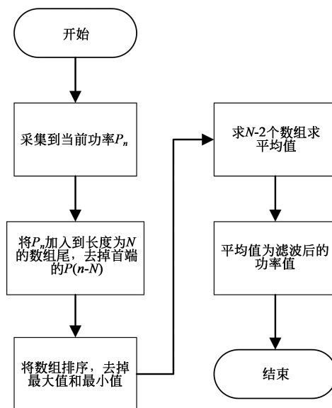
图5 数字滤波流程图
