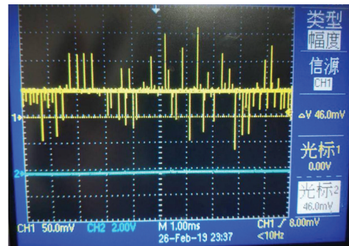
图 7 传统放大滤波后信号
