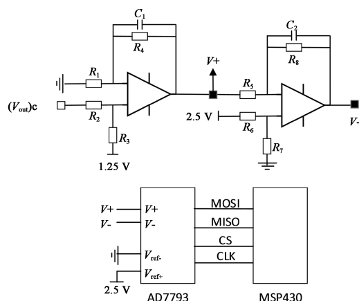
图3 单端转差分采集电路图
