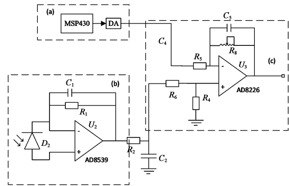
图 2 光照前端采集电路图
