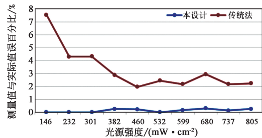
图 8 面光源不同强度下检测数据及误差分布图
