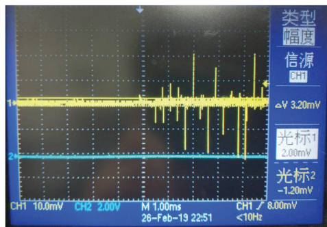
图 6 本设计放大滤波后信号
