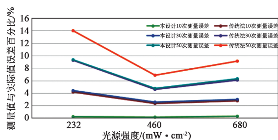
图 9 面光源不同强度下多次检测数据误差分布图
