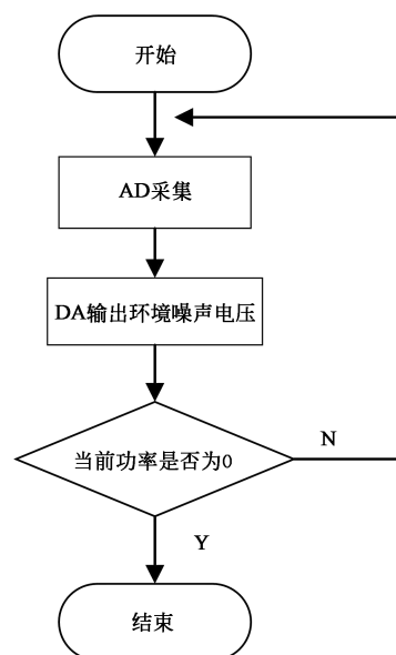
图4 校零流程图
