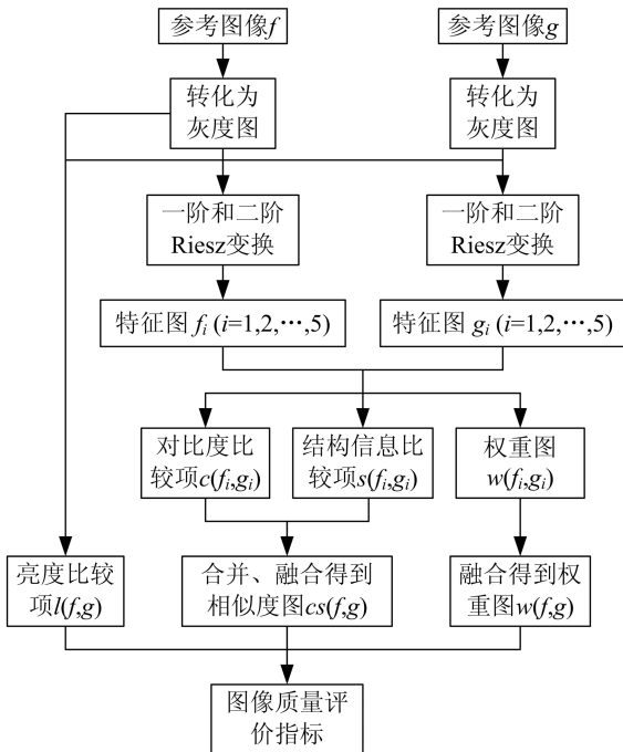
图 3 本文所提算法的实现框图
