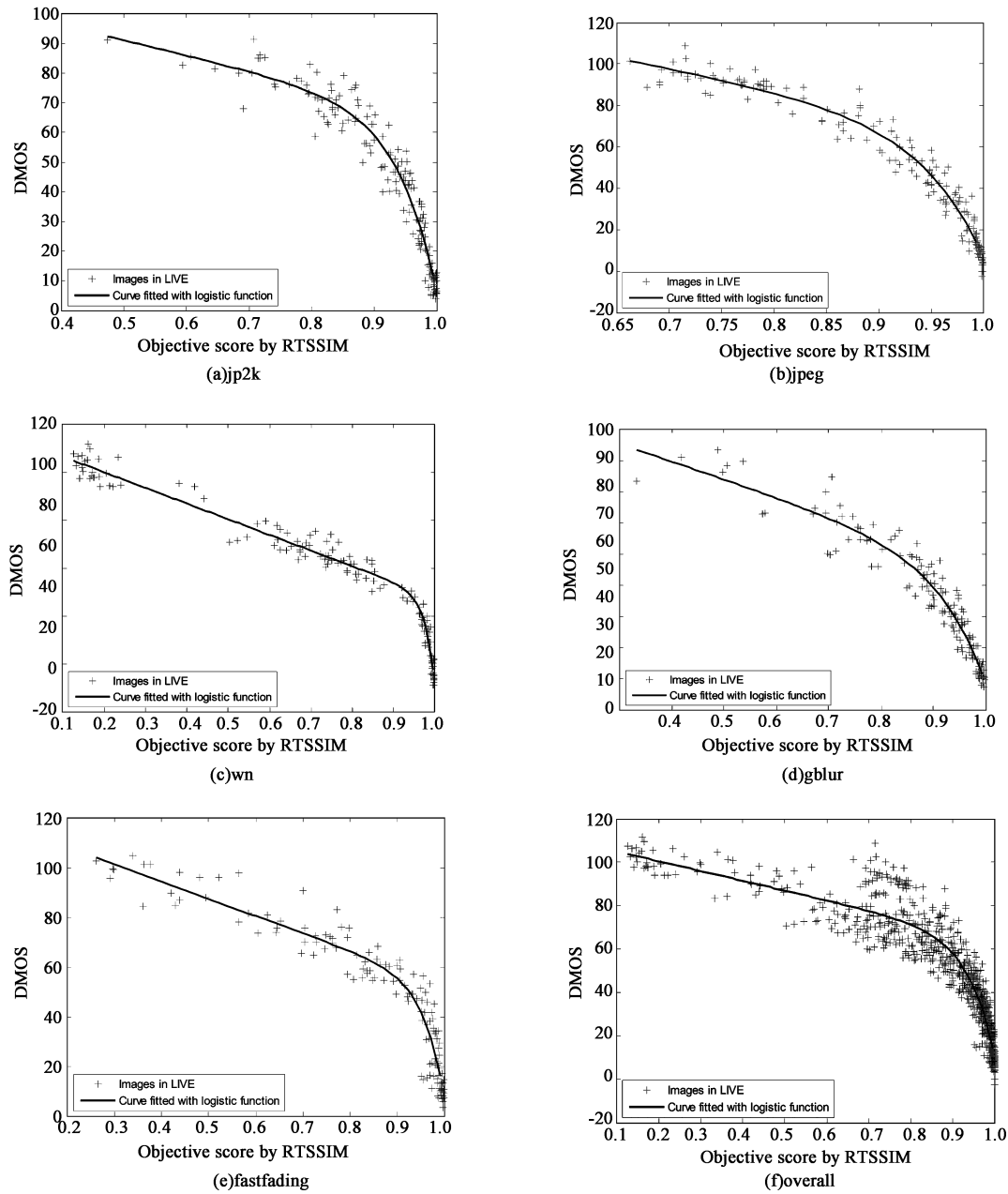
图 4 本文所提出的图像质量评价方法(RTSSIM)与主观 DMOS 的曲线拟合图
