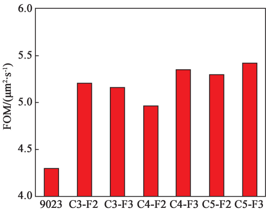
图 5 6 种液晶化合物溶于商品液晶材料 9023 后响应性能
