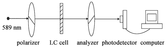
图 2 测定 \Delta n 值和响应时间的光路图
