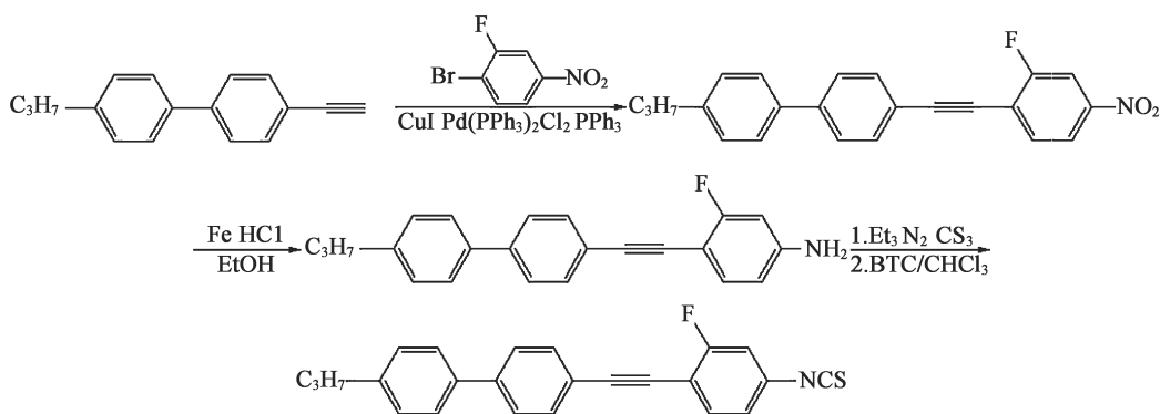
图 1 4'-正丙基-2-氟-4-异硫氰酸酯-苯基二苯乙炔的合成过程
