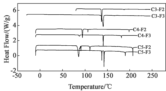
图 3 6 种液晶化合物的差热分析谱图
