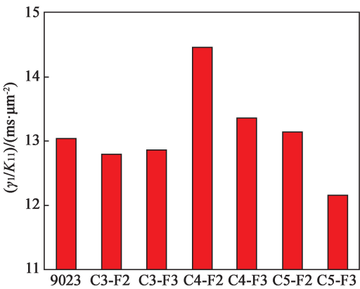
图 4 6 种液晶化合物溶于商品液晶 9023 后的黏弹系数
