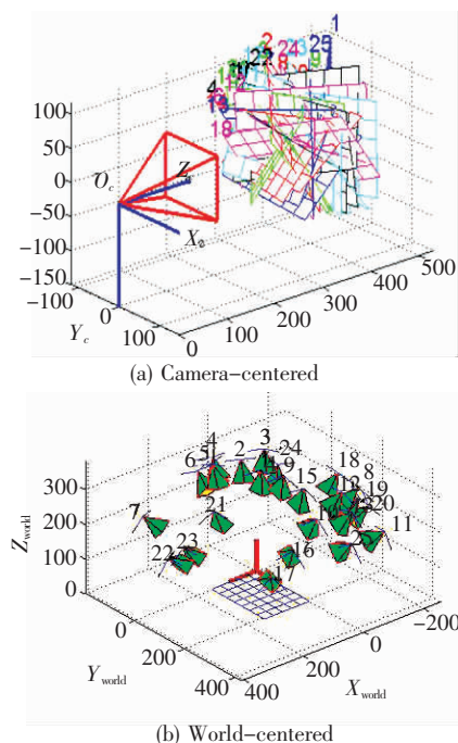
图 5 三维空间模型
