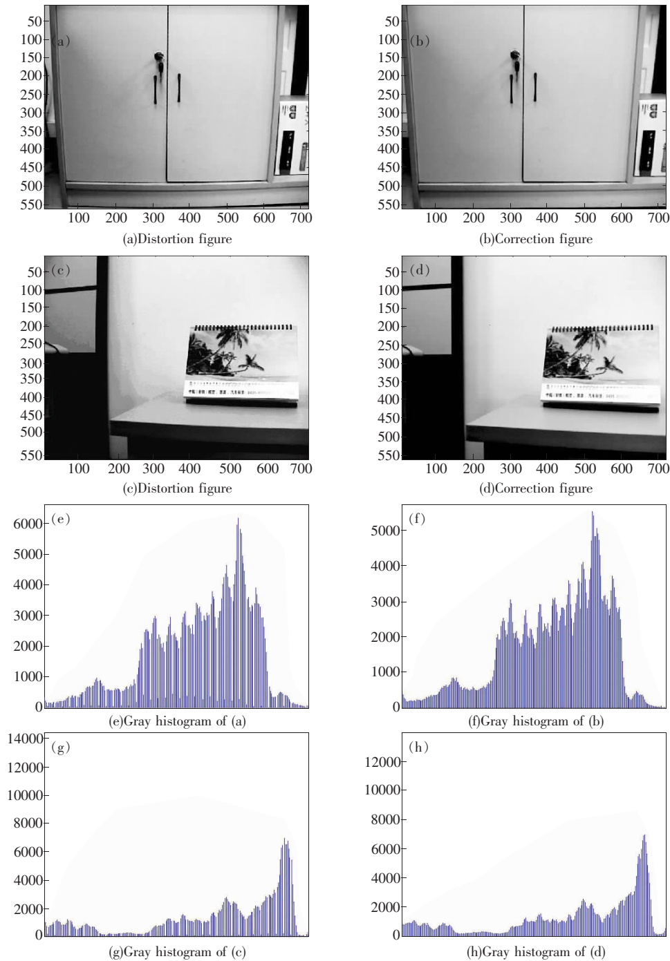
图 7 校正前后实物图和其灰度直方图对比
