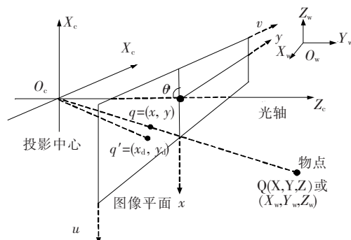
图 1 摄像机标定模型
