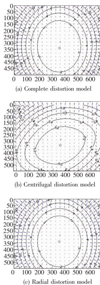
图 6 畸变模型中的畸变成分
