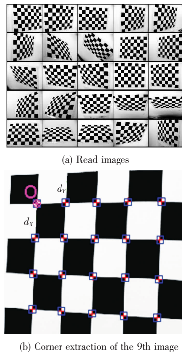
图3 读入图像与角点提取
