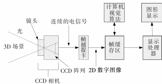
图2 图像采集与处理的系统装置
