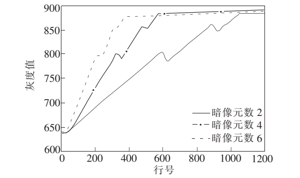
图 5 校正速度与 CCD 暗像元个数的关系
