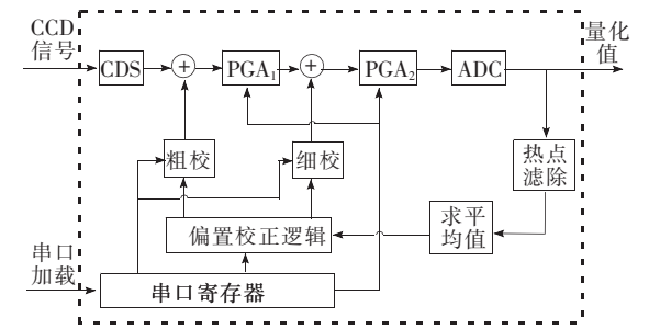
图 1 XRD98L59 内部结构 Fig. 1 Architecture of XRD98L59
