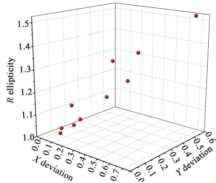
图 10 椭圆率对圆心坐标偏差的影响
