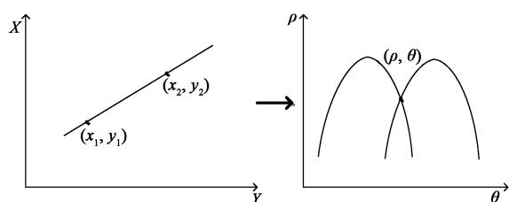
图 5 直角坐标到极坐标的转换。(a)直角坐标;(b)极坐标。
